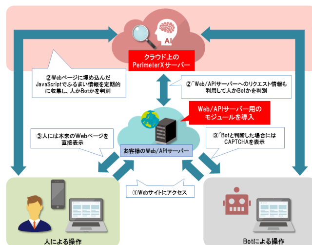
図 1. 「PerimeterX Bot Defender」のイメージ図
