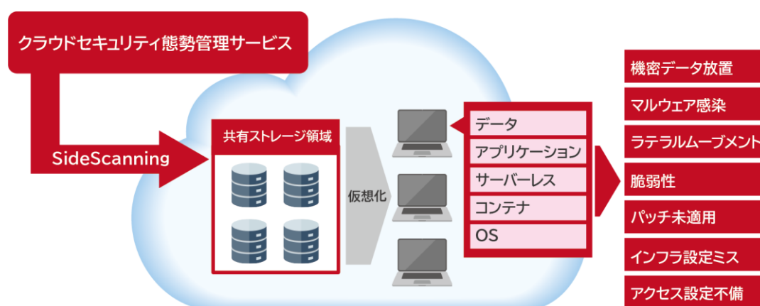
図1: SideScanningによりエージェントソフトを使わずセキュリティリスクを検出
